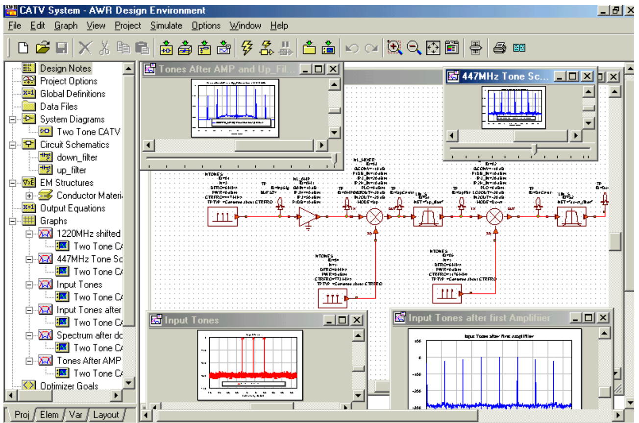
Рис. 10. Схема VSS анализа линии связи абонентского телевидения
