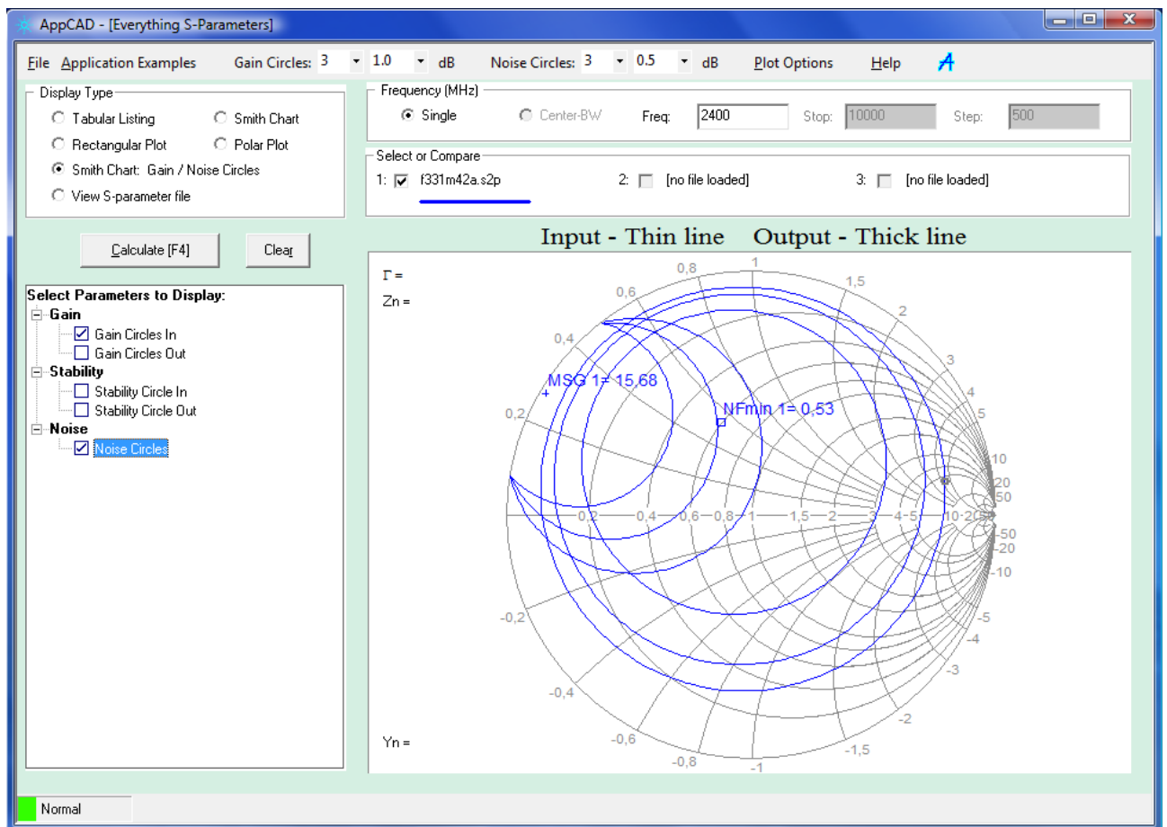
Рис. 12. Интерфейс программы AppCAD, с электронной диаграммой Смита
