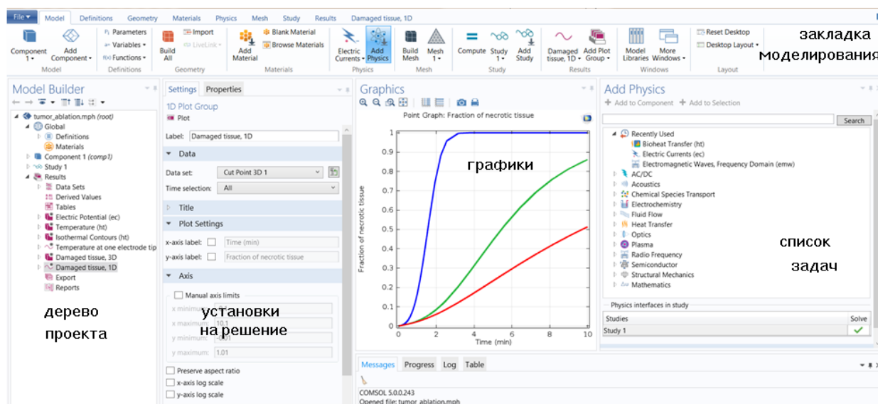
Рис. 24. Общий интерфейс программы COMSOL Multiphysics
