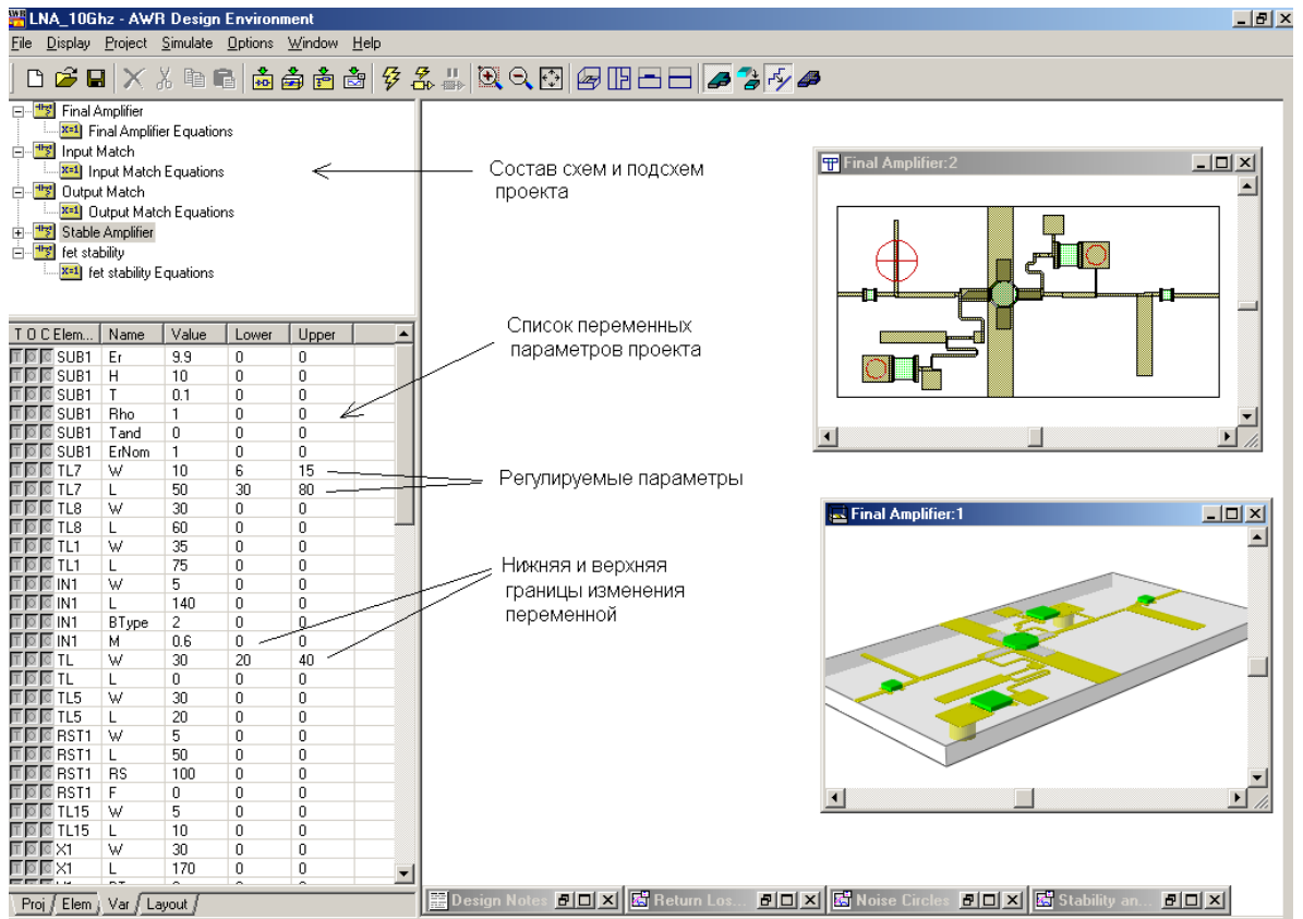
Рис. 11. Интерфейс программы MWO AWR
